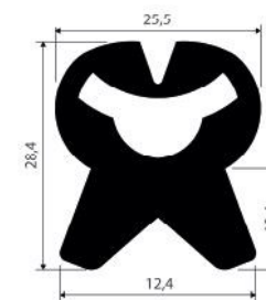
Perfil en caucho EPDM Ref: 14/2
