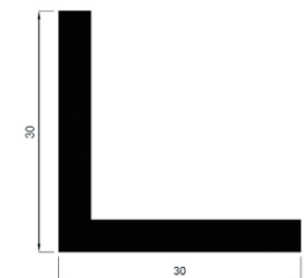
Perfil goma forma L 30 x 30
