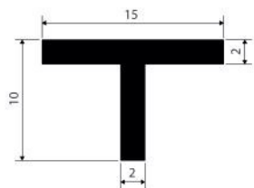
Perfil en caucho EPDM FORMA T
