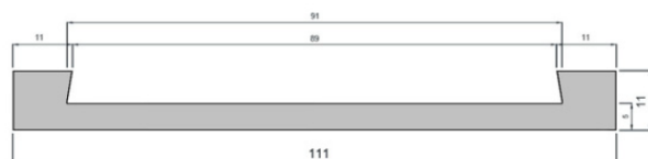
Perfil en caucho EPDM Blanco
