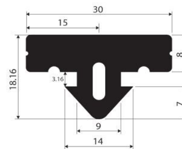
Perfil en caucho EPDM Ref: 30 x 18,16
