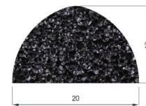
Perfil caucho esponjoso Media caña 20 x 12
