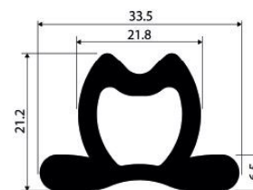
Perfil en caucho
