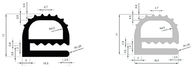
Perfil en silicona gris y caucho EPDM negro
