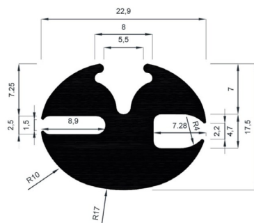
Perfil en caucho EPDM Ref: 105 + junquillo
