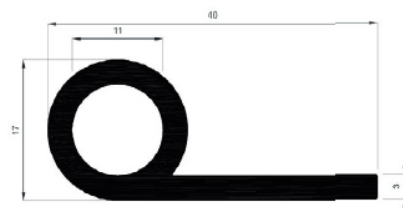
Perfil en caucho EPDM Ref: 19 forma 9
