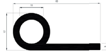
Perfil en caucho EPDM Ref: 19 forma 9
