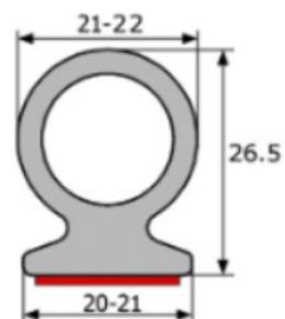
Perfil de caucho esponjoso ref: Omega
