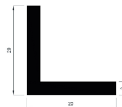
Perfil goma forma L 20 x 20
