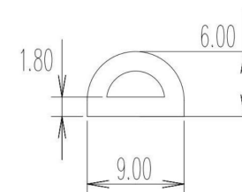
Perfil caucho esponjoso Media caña 9 X 6 c/adh.
