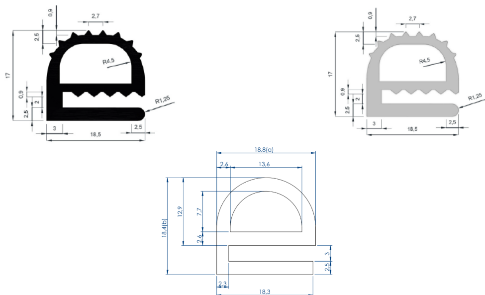
Perfil en silicona gris y caucho EPDM negro FORMA e
