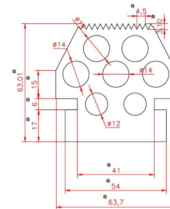
Perfil en caucho EPDM REF: CB -65
