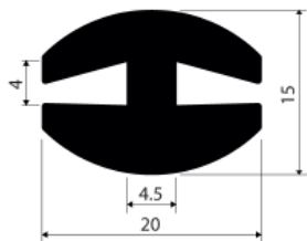
Perfil en caucho EPDM Ref: Forma H
