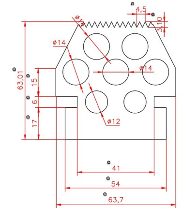
Perfil en caucho EPDM REF: CB -65
