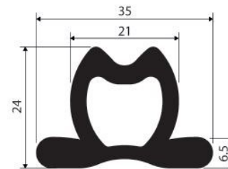
Perfil en caucho EPDM Ref: 14
