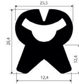
Perfil en caucho EPDM Ref: 14/2
