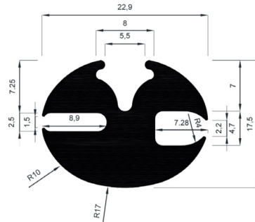
Perfil en caucho EPDM Ref: 105 + junquillo
