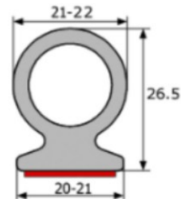
Perfil de caucho esponjoso ref: Omega
