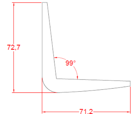
Perfil goma forma L 70 x 70
