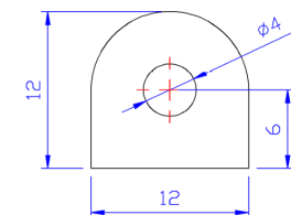
Perfil en silicona Ref: 12x12D
