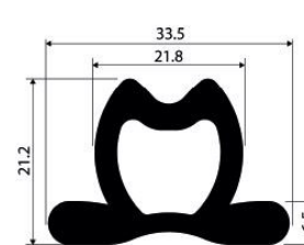
Perfil en caucho
