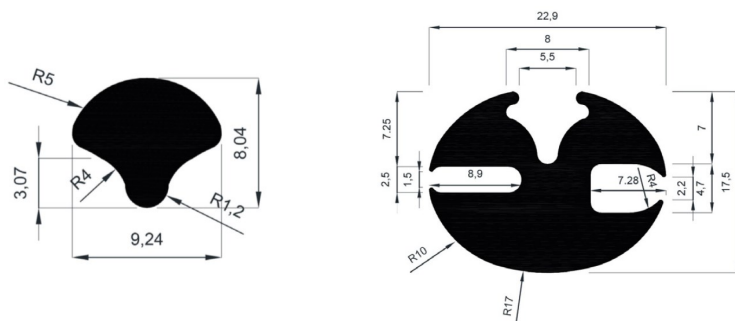
Perfil en caucho EPDM Ref: 105 + junquillo
