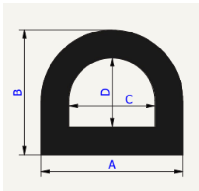
Perfil DEFENSA FORMA D
