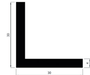
Perfil goma forma L 30 x 30
