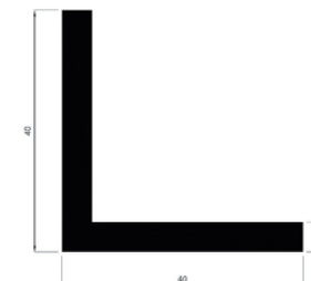
Perfil goma forma L 40 x 40
