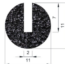
Perfil en caucho esponjoso Ø 12
