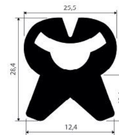
Perfil en caucho EPDM Ref: 14/2
