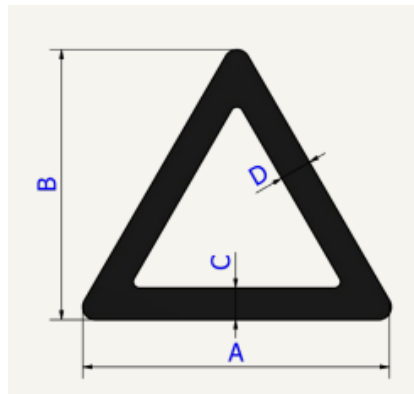
Perfil DEFENSA FORMA TRIANGULAR
